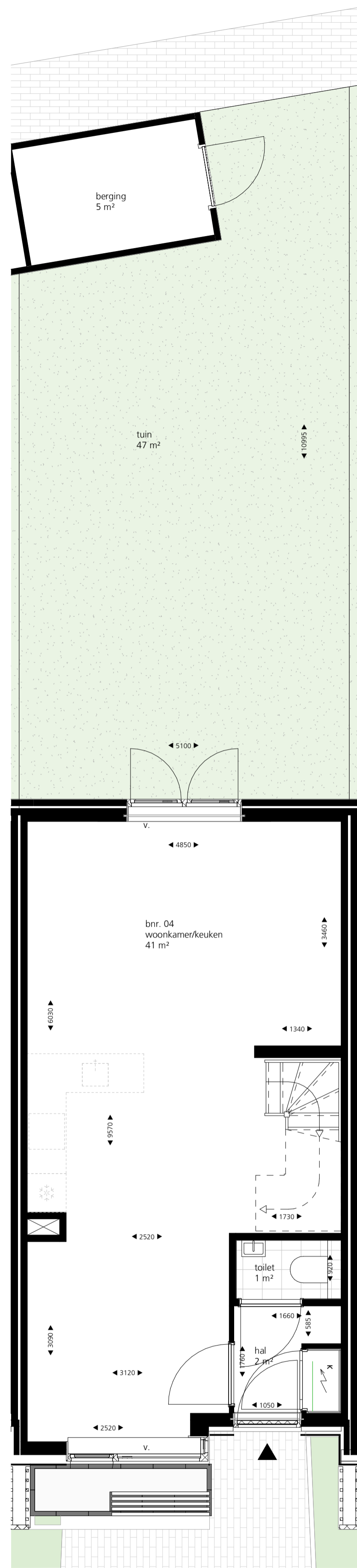
begane grond
