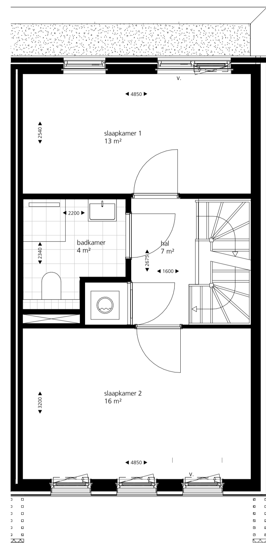
eerste verdieping
