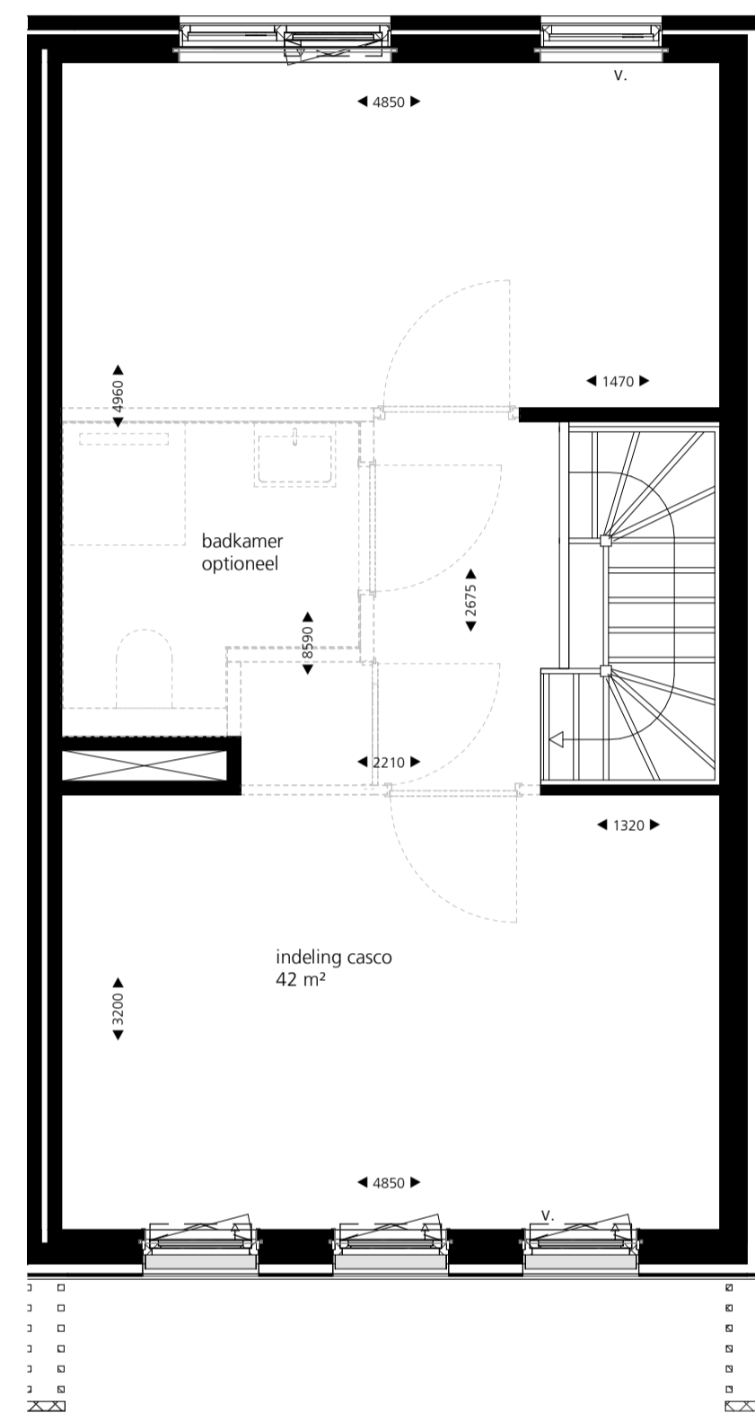
tweede verdieping
