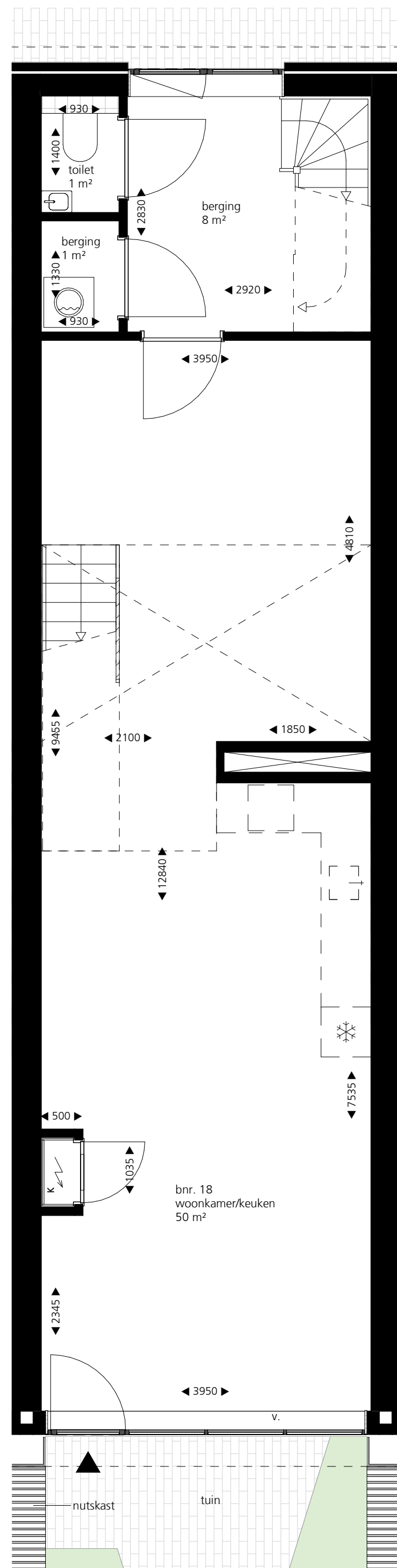
begane grond
