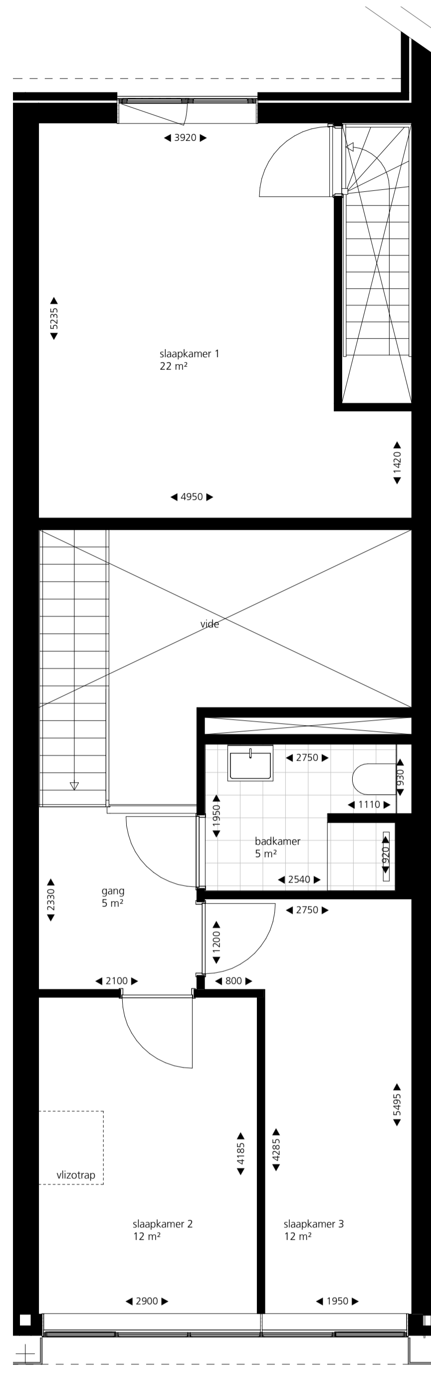
eerste verdieping
