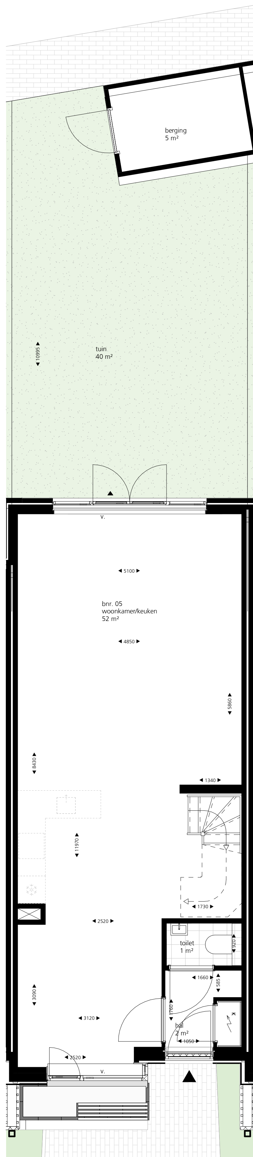
begane grond
