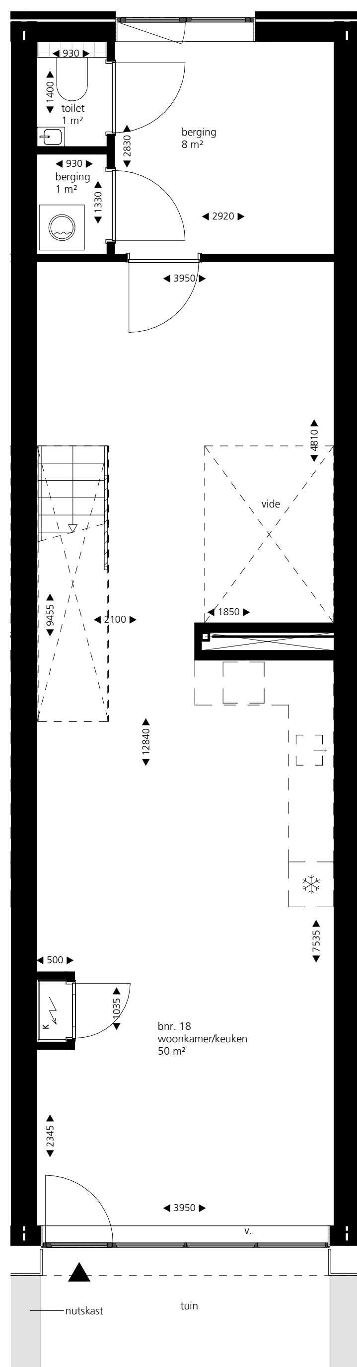
begane grond
