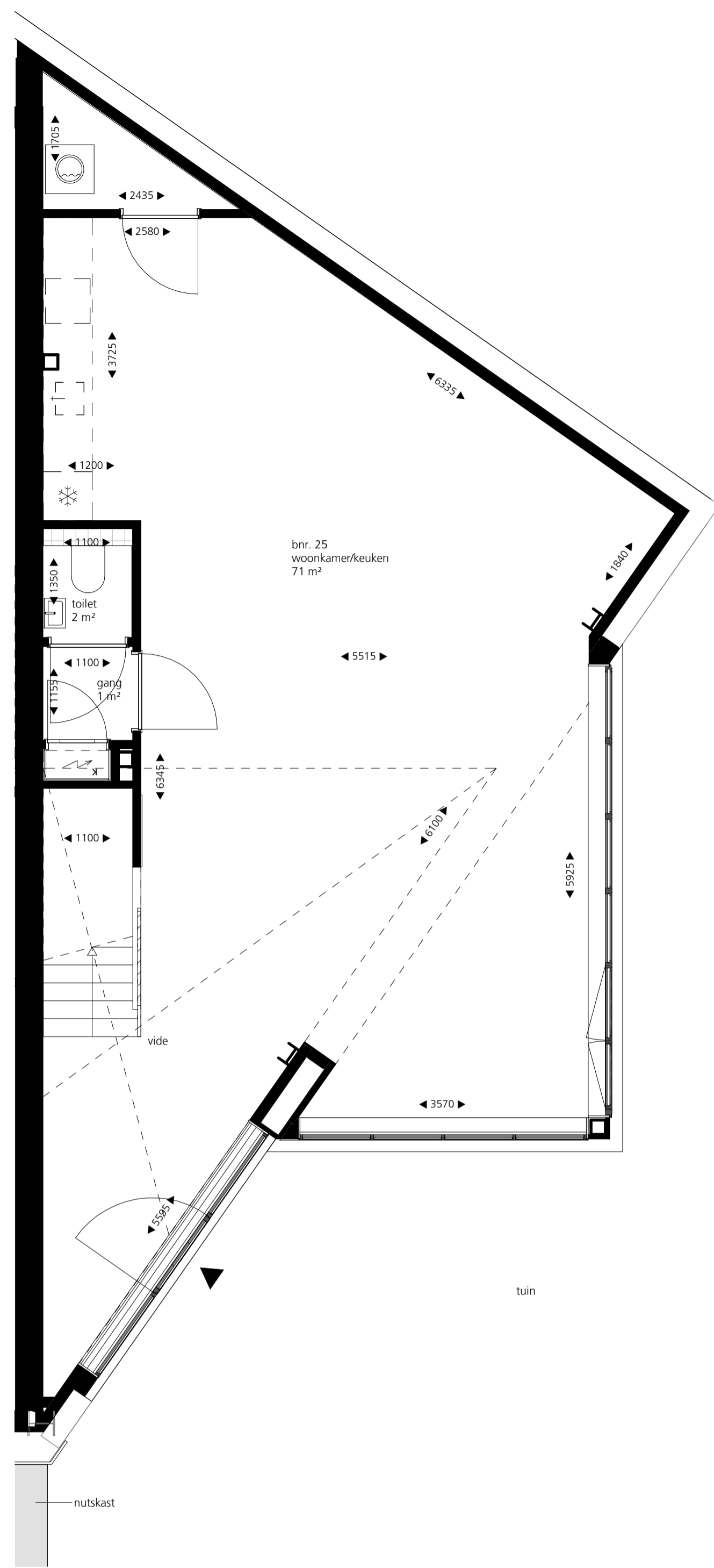
begane grond
