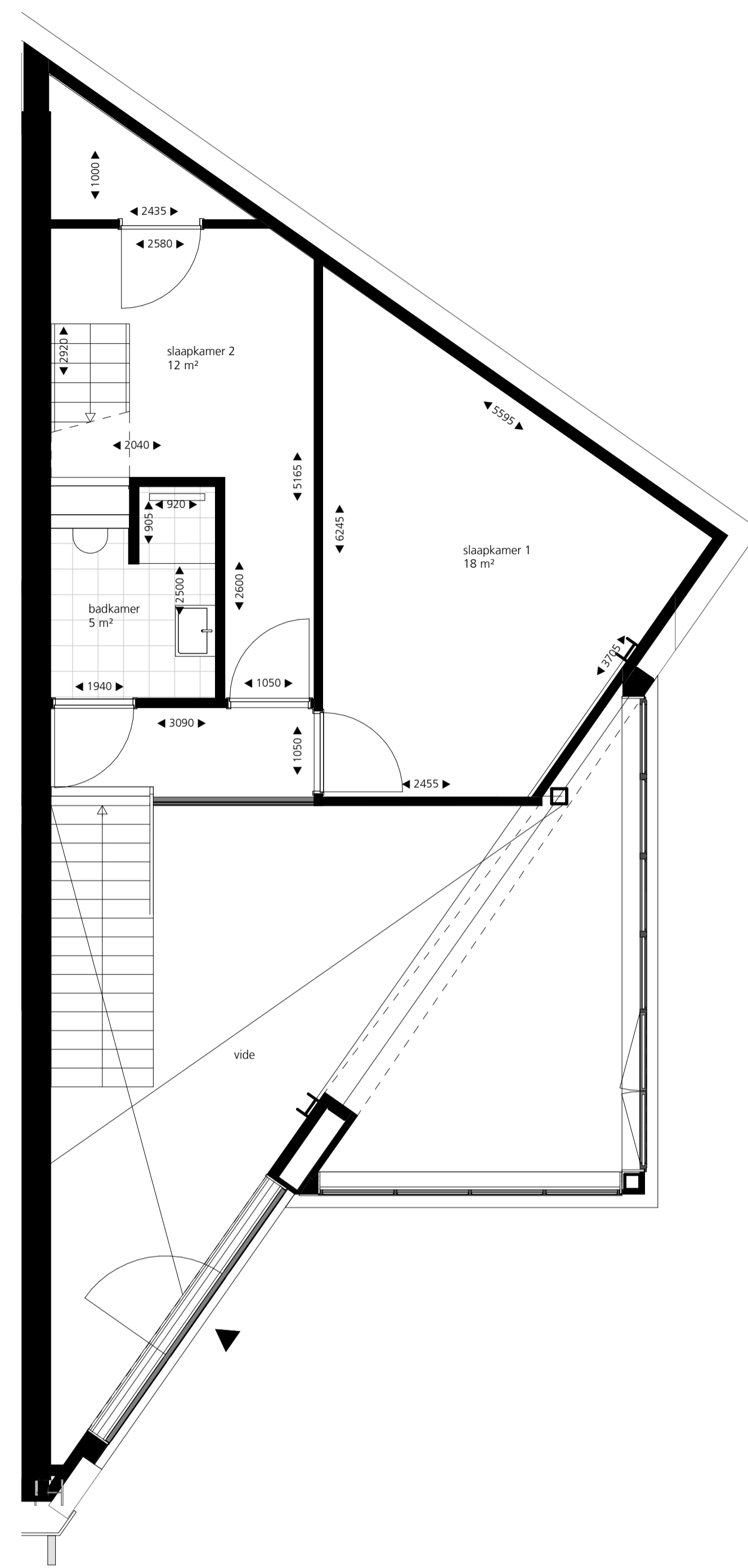
eerste verdieping
