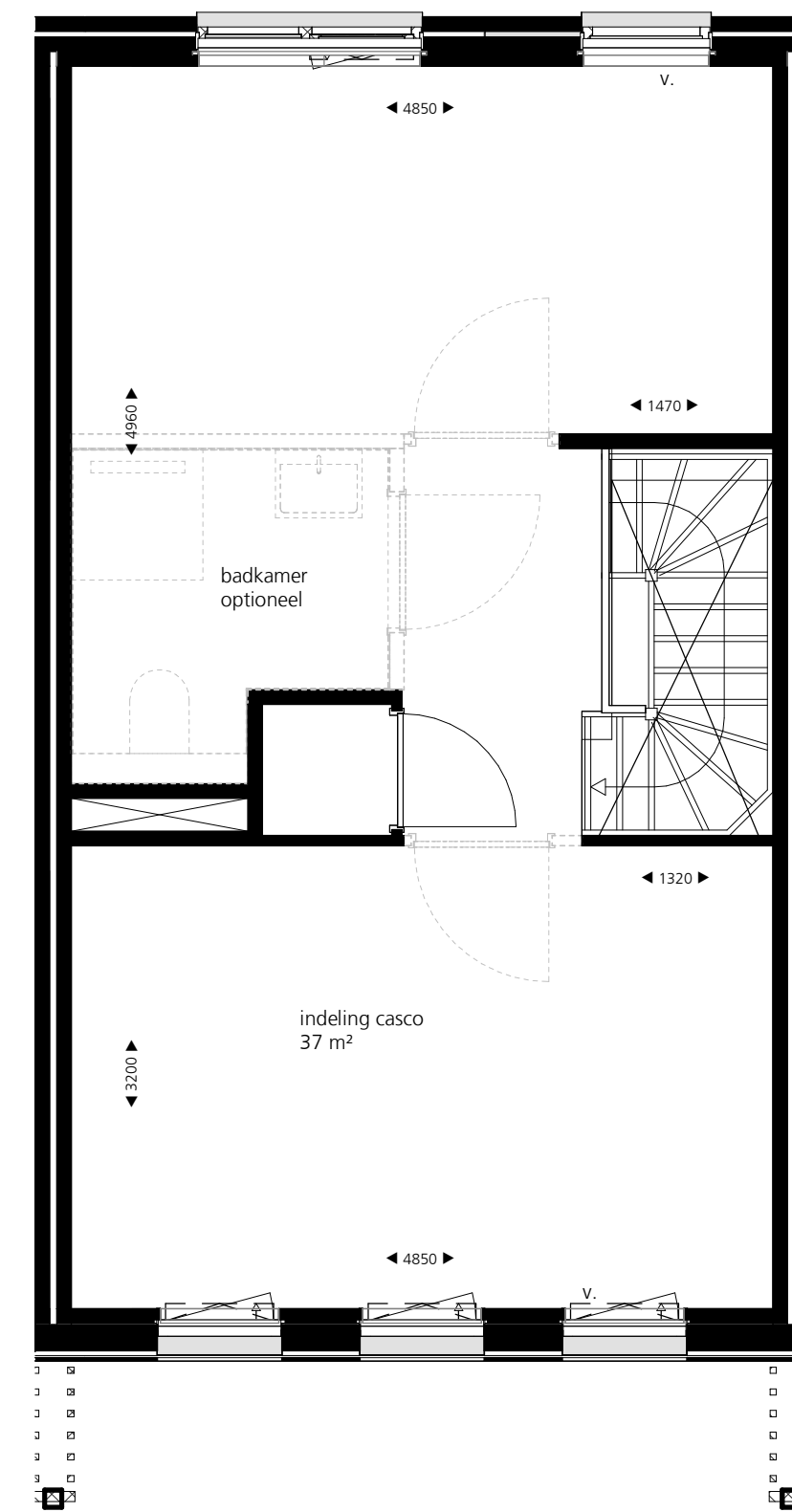
tweede verdieping
