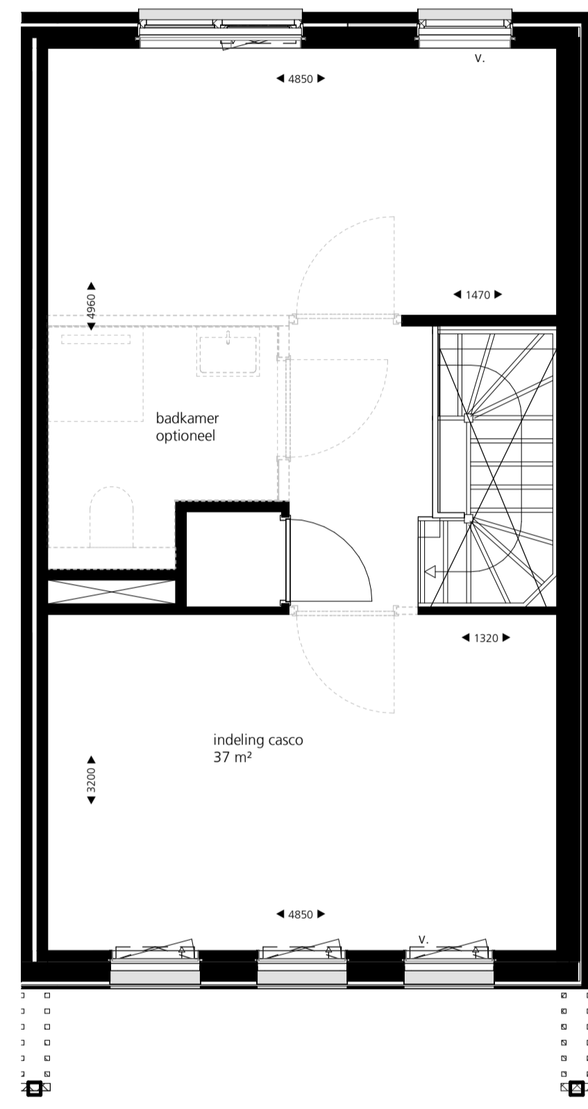
tweede verdieping
