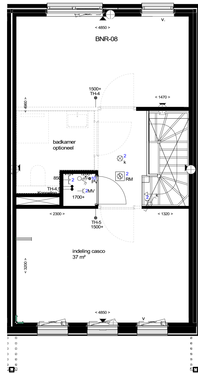
tweede verdieping
