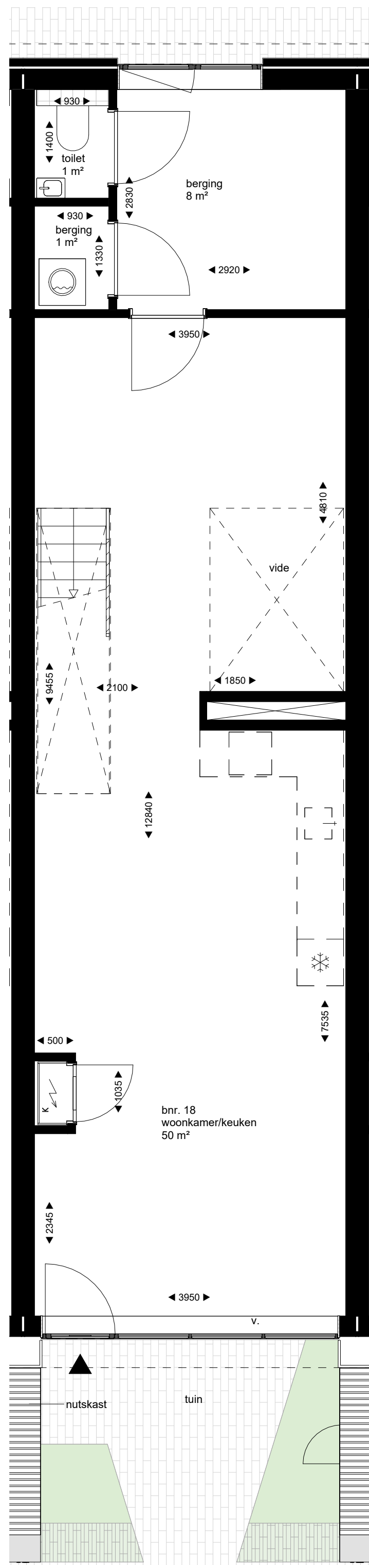
begane grond
