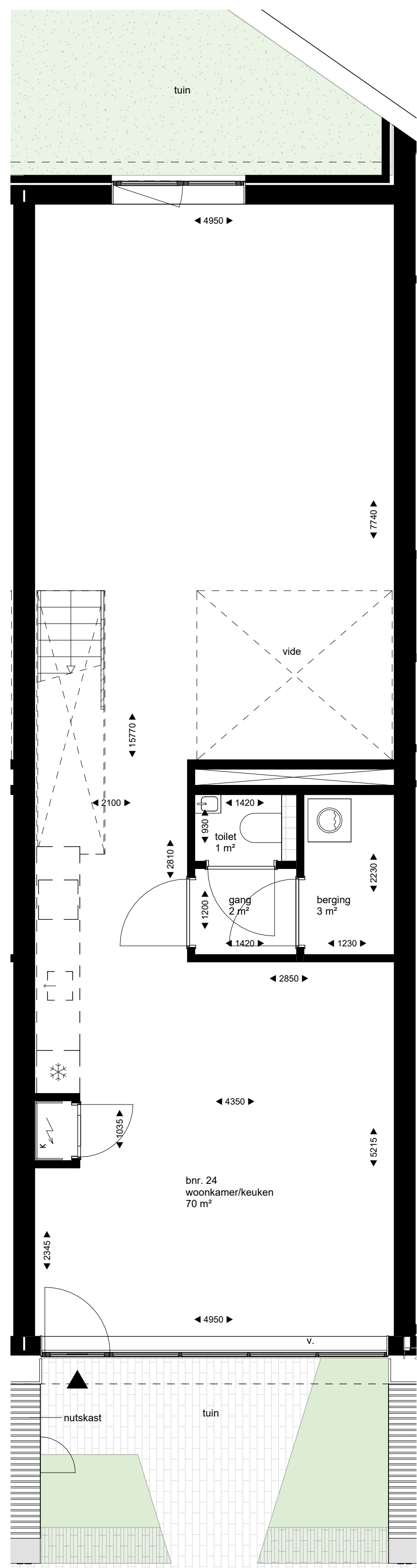
begane grond
